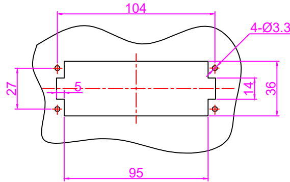
面板开孔图
